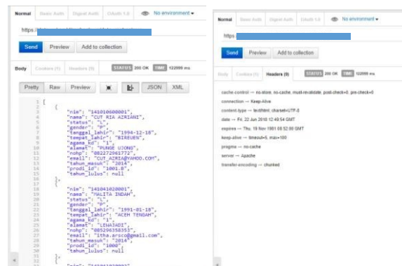
Gambar 4. Tampilan aplikasi postman REST client pengujian REST API data mahasiswa
