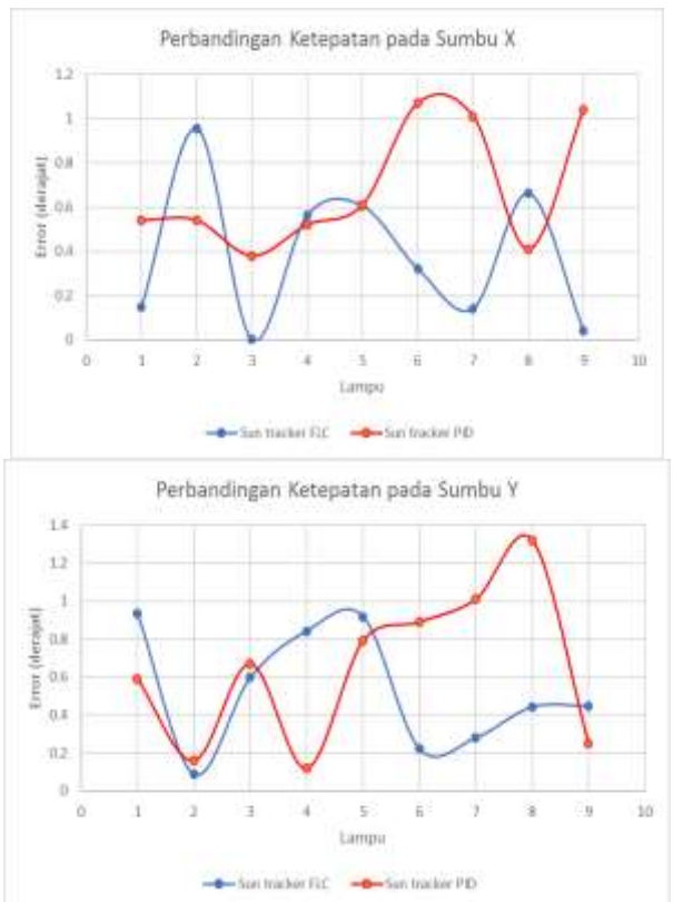
Gambar 8. Perbandingan Ketepatan Sudut Sumbu X dan Sumbu Y
