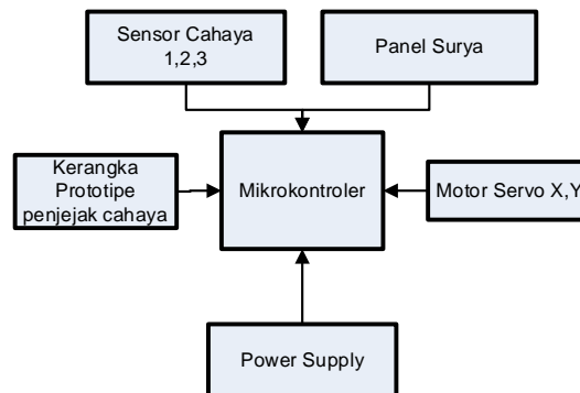
Gambar 3. Struktur Hardware Penjejak Cahaya
