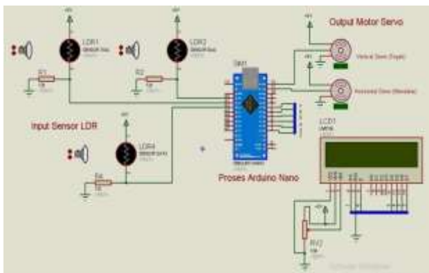
Gambar 2. Rangkaian Konfigurasi Sistem Penjejak Cahaya
