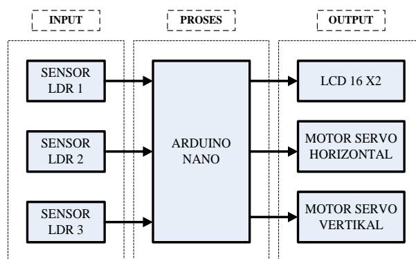
Gambar 1. Blok Diagram Sistem Penjejak Cahaya
