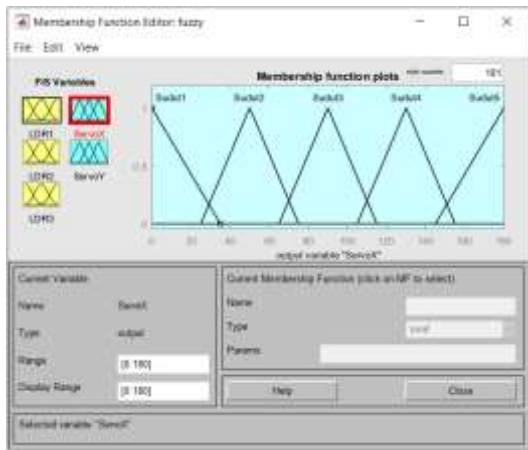
Gambar 4. Membership input dan output FLC
