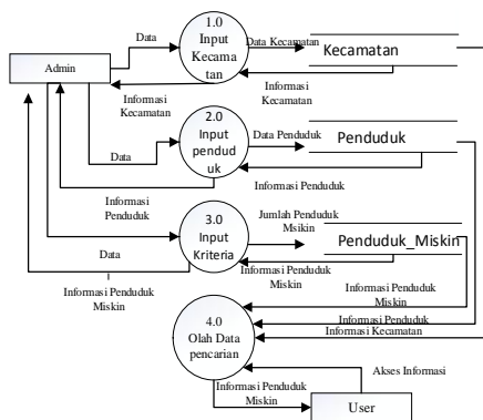
Gambar 3. Diagram Overview atau Level 1 SIG
