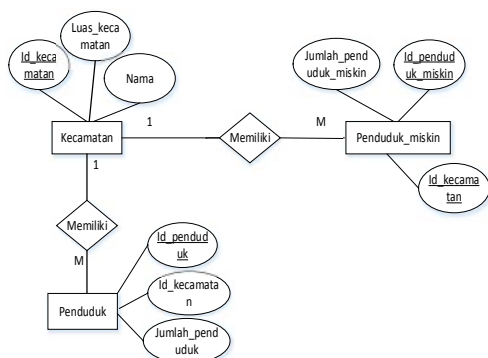
Gambar 8. ERD SIG
