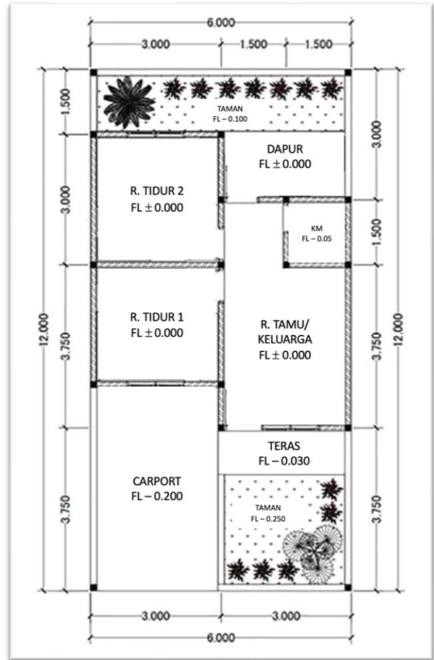
Gambar 4.1. Denah Rumah Tipe 36 Perumahan Sanggamara
